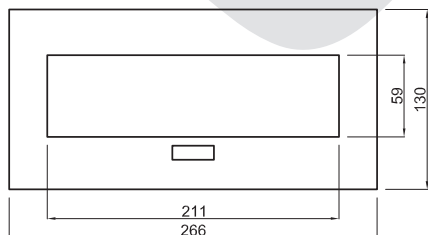
wymiary rozgąłęziacza
